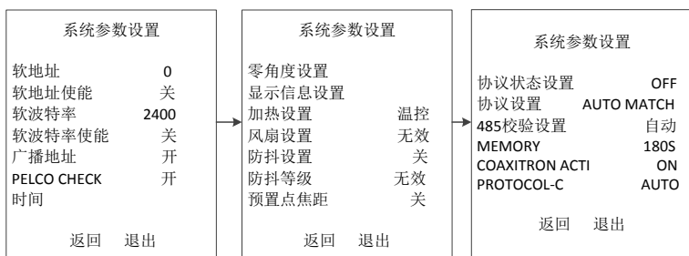
图4-1 系统参数设置
