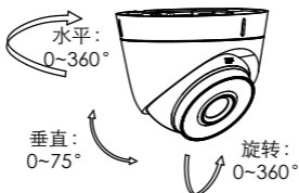
图3-5 角度调节
