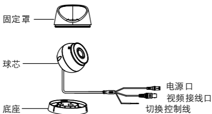
图2-1 I型摄像机概览图
